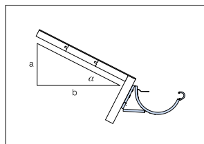
Lindab SSK ställbar snäppkrok
