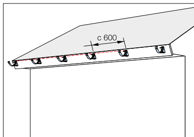
Fäst resten av krokarna med cc 600 mm längs snöret.
