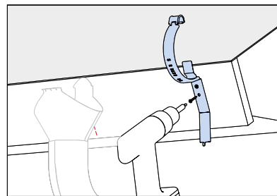
Fäst kroken till höger om markeringen för stupröret 2,5 mm ovanför den nedre kroken.
