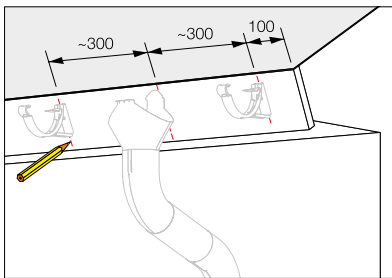
Märk ut placeringen för SSK ställbara snäppkrokar runt stupröret.
