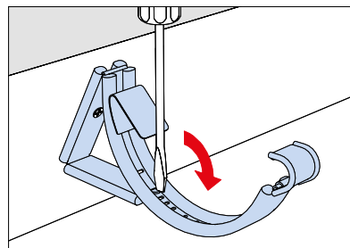
Använd skruvmejsel för att vika fliken framåt för liten vinkel och bakåt för \alpha \geq 22^\circ .
