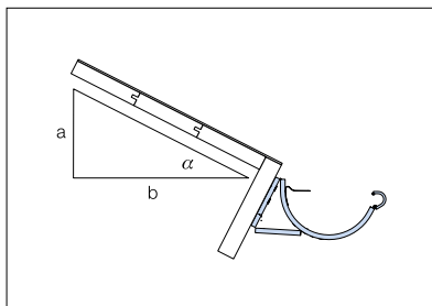
Mät takvinkeln och justera krokarna därefter.
