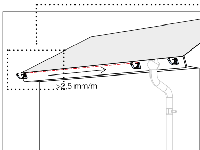
Fäst den övre kroken på takfotens andra sida. Rörlutningen ska vara 2,5 mm/m.
