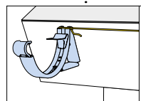
Spänn ett snöre mellan hög och låg krok. På så sätt blir det lättare att montera resten av krokarna.
