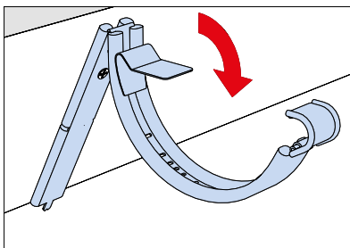
SSK ställbara snäppkrokar kan justeras för olika takvinklar.
