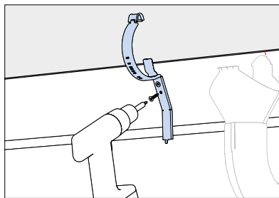
Fäst den nedre kroken 300 mm till vänster om markeringen för stupröret.
